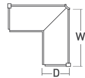
SP - 310 B 1384W x 460D x 1489H mm.
