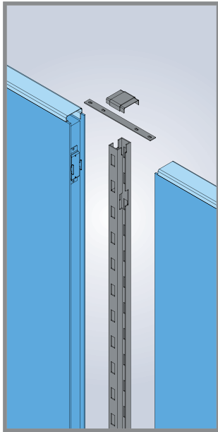
UPRIGHT
