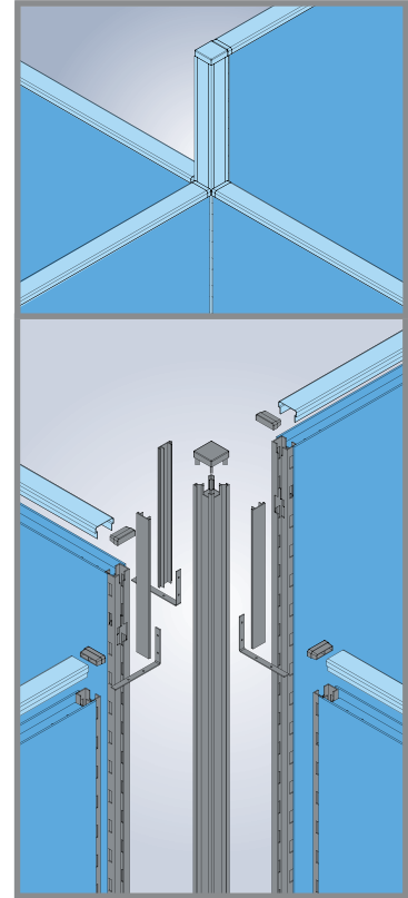
"+" TYPE CORNER PIECE (D)
